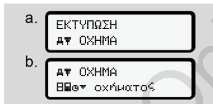
Εικ. 93: Αλληλουχία μενού εκτύπωσης - Πληροφορίες καρτών ταχογράφου
